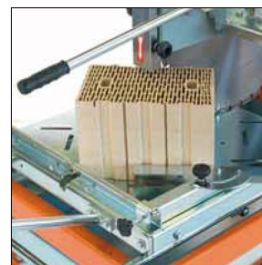
Winkelanschlag 0 – 180°
